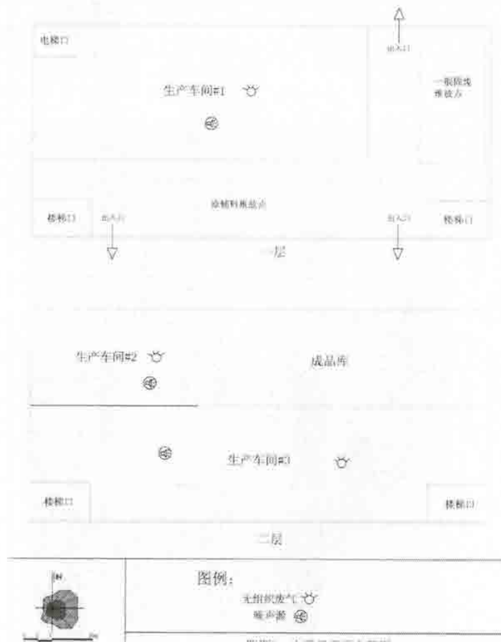
图 3.1-3 项目厂区平面图
